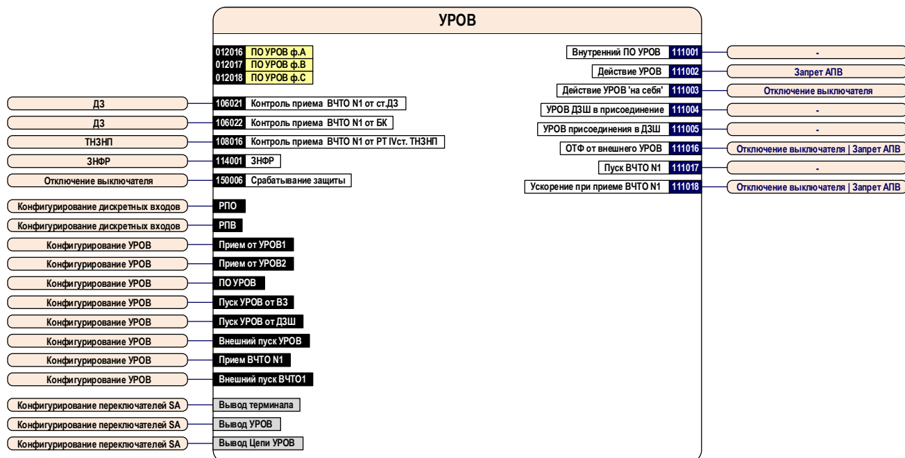
Рисунок 9. Блок – схема узла УРОВ
