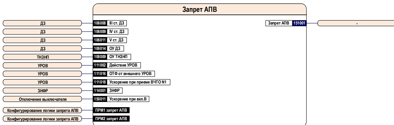
Рисунок 15. Блок – схема узла запрета АПВ выключателя
