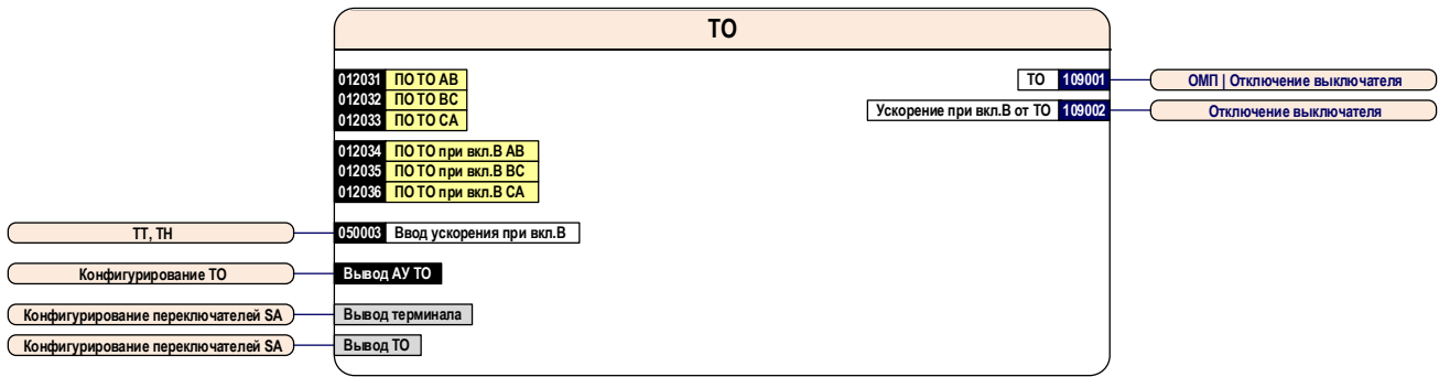
Рисунок 8. Блок – схема узла ТО
